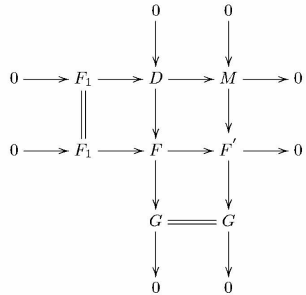
图 5 D \longrightarrow F 和 D \longrightarrow M 的推出
