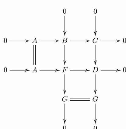
图 3 B \longrightarrow C 和 B \longrightarrow F 的推出
