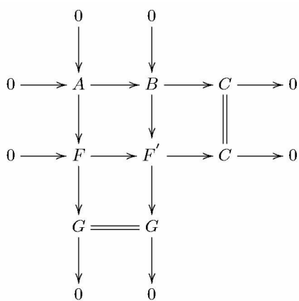
图 2 A \longrightarrow B 和 A \longrightarrow F 的推出
