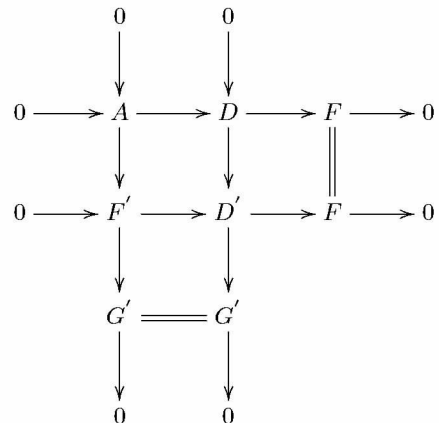
图 7 A \longrightarrow F' 和 A \longrightarrow D 的拉回
