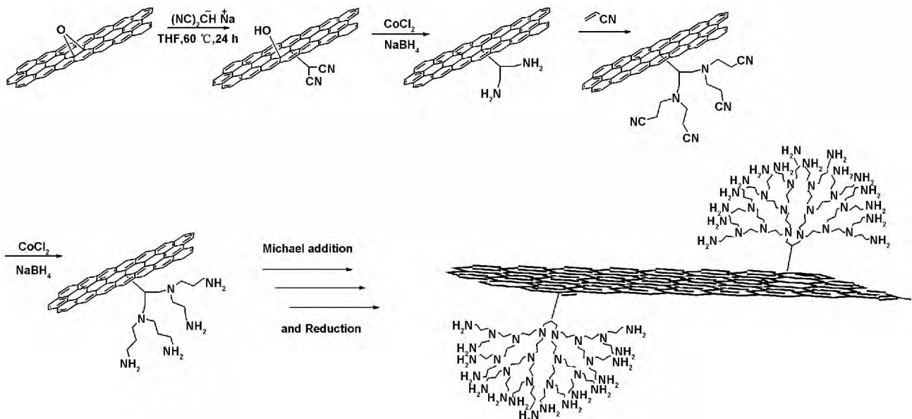
图1 石墨烯表面接枝聚丙烯亚胺树状大分子的合成路线 [25]
